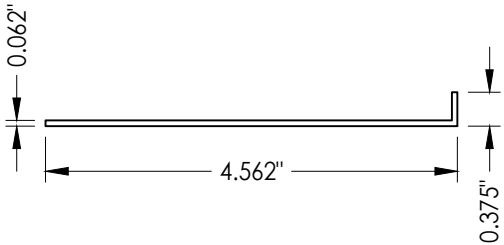
4 SILL PAN
