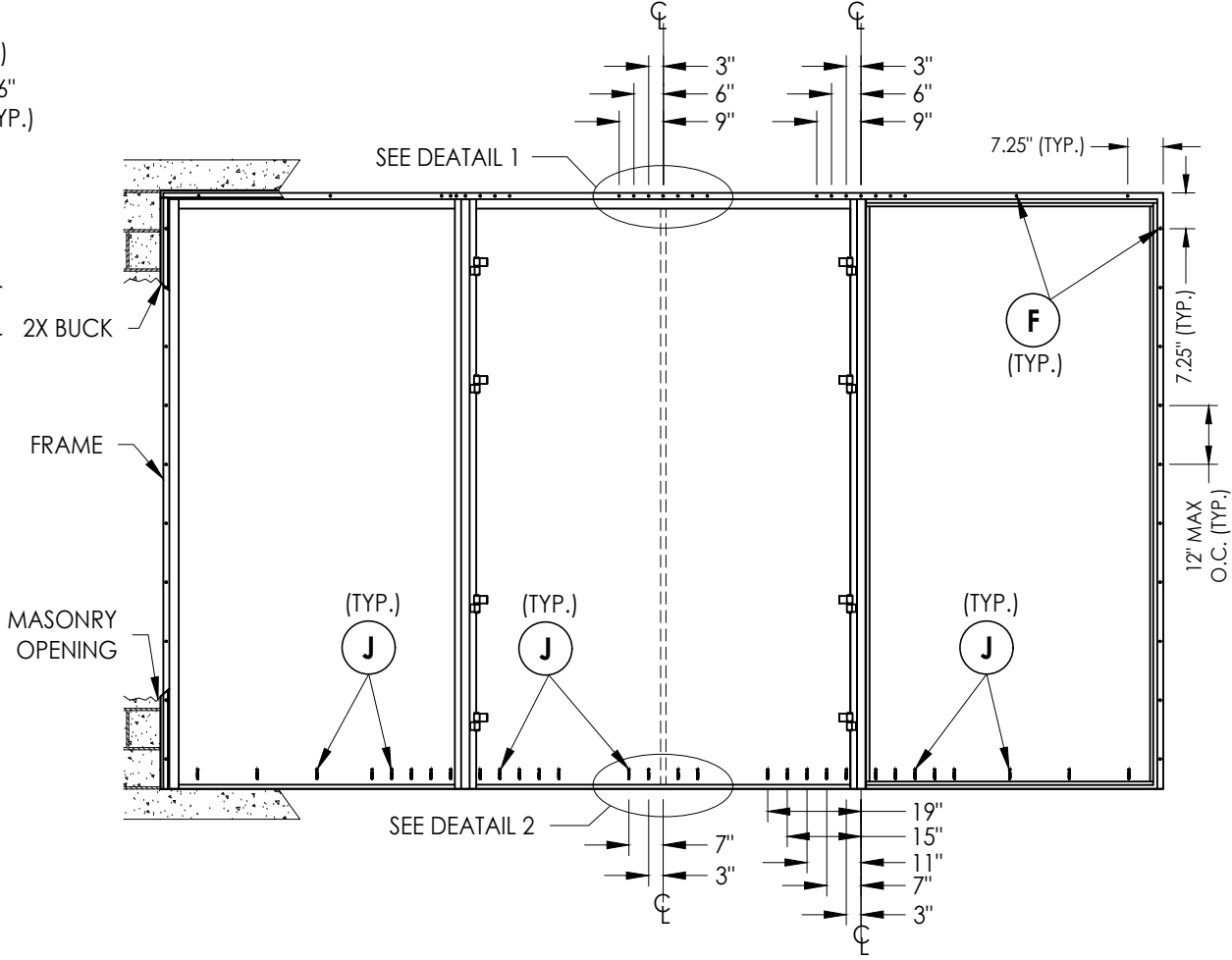
FIN ANCHORING
